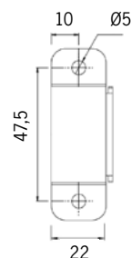
Fästbygel avslut 1025668
